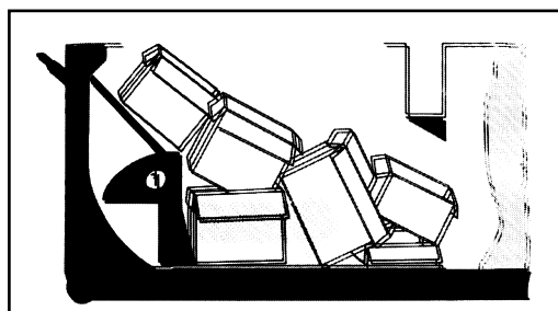
1 Det selvrensende vendesetempelet vist i den ytterste, helt tilbaketrukne stillingen.
